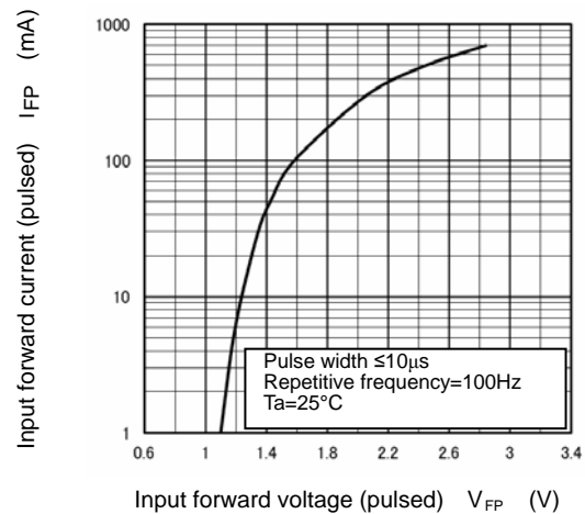
I_{FP} - V_{FP}
