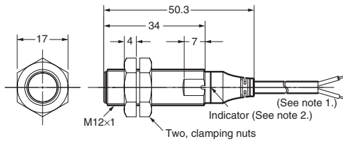
E2AU-M12KS04-WP-□□
