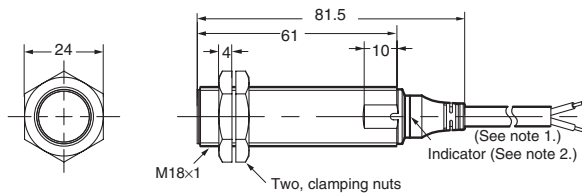
E2AU-M18LS08-WP-□□
