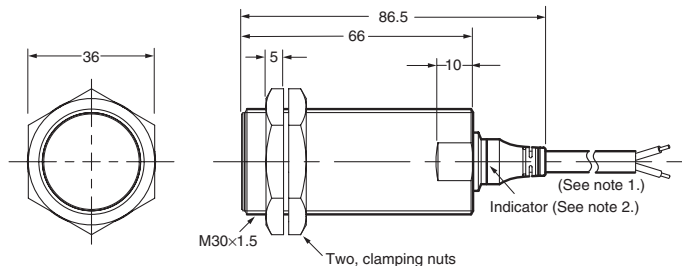
E2AU-M30LS15-WP-□□
