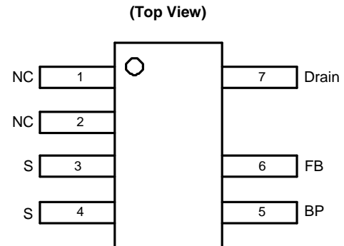
SO-7
