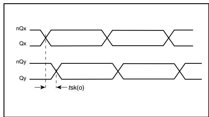
Output Skew
