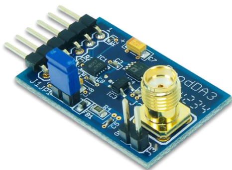
The PmodDA3.
