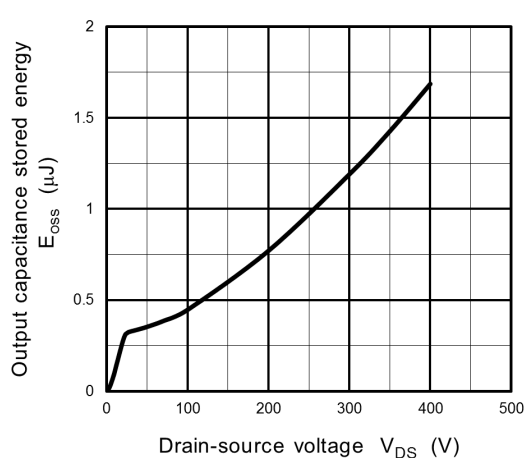
Fig. 8.10 E_{OSS} - V_{DS}
