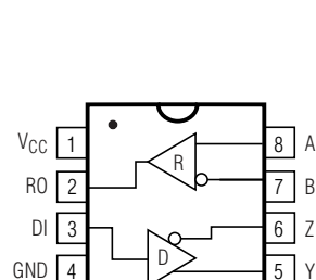
DIP/SO
