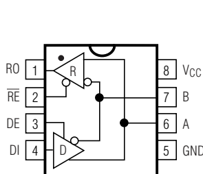
DIP/SO
