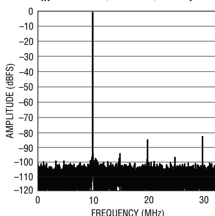
LTC2258-14: 8k Point FFT, f_{IN} = 140\text{MHz} , -1\text{dBFS} , 65\text{Mps}
