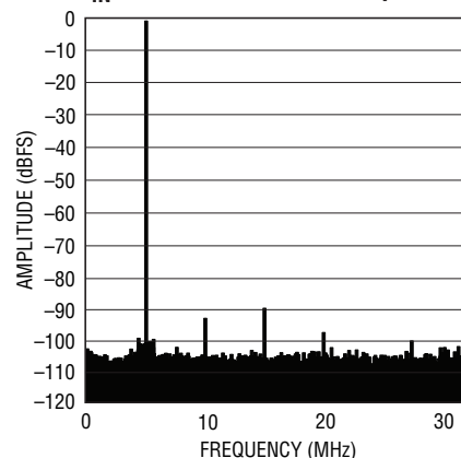
LTC2258-14: 8k Point FFT, f_{IN} = 5\text{MHz} , -1\text{dBFS} , 65\text{Mps}
