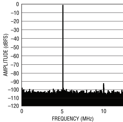
LTC2256-14: 8k Point FFT, f_{IN} = 5\text{MHz} , -1\text{dBFS} , 25\text{Mps}
