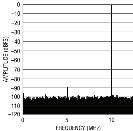
LTC2256-14: 8k Point FFT, f_{IN} = 140\text{MHz} , -1\text{dBFS} , 25\text{Mps}
