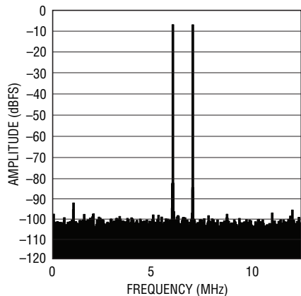
LTC2256-14: 8k Point 2-Tone FFT, f_{IN} = 68\text{MHz} , 69\text{MHz} , -1\text{dBFS} , 25\text{Mps}
