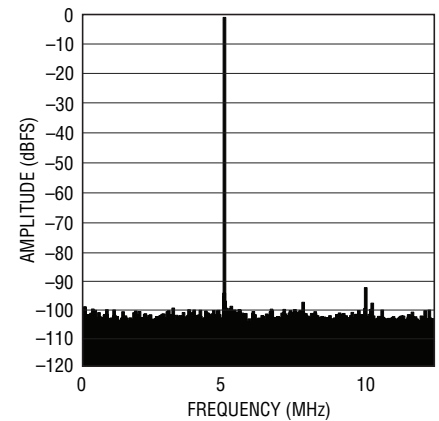
LTC2256-14: 8k Point FFT, f_{IN} = 70\text{MHz} , -1\text{dBFS} , 25\text{Mps}
