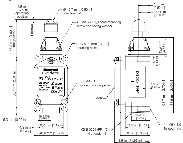
Figure 9. SZL-WL-I
