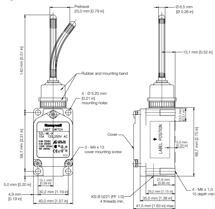
Figure 11. SZL-WL-K
