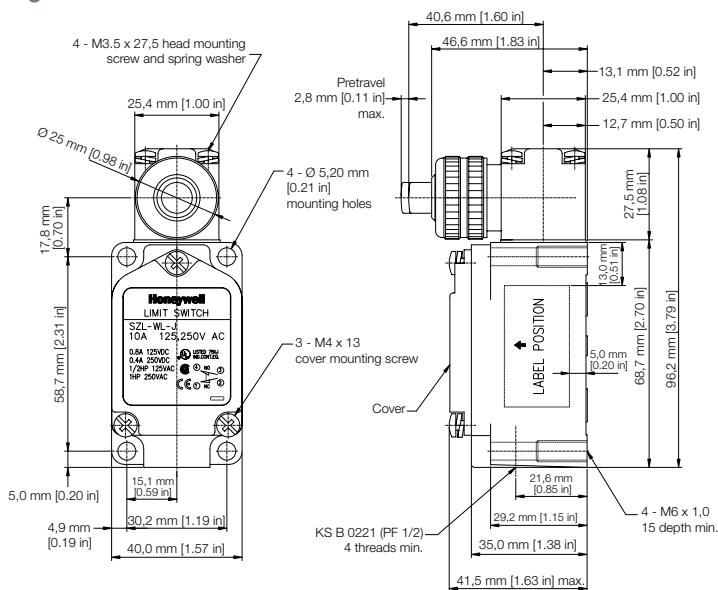
Figure 10. SZL-WL-J
