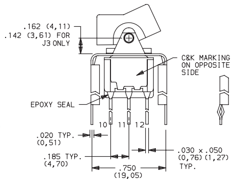
7401J1_BE2 4PDT
