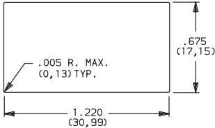
J37 Actuator
