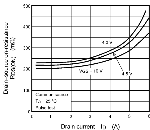
Fig. 7.4 R_{DS(ON)} - I_D
