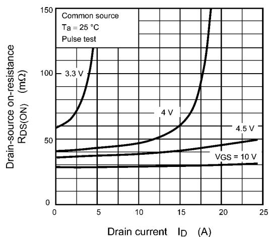
Fig. 8.4 RDS(ON) - ID
