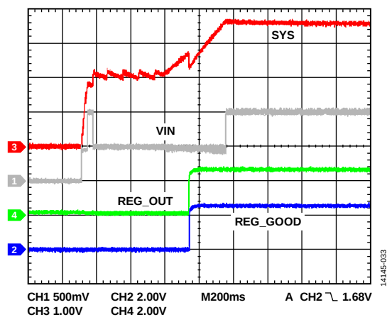
Figure 35. REG_GOOD Function
