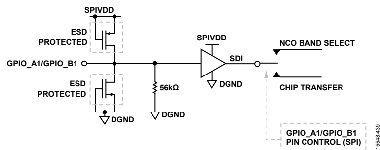
Figure 41. GPIO_A1/GPIO_B1
