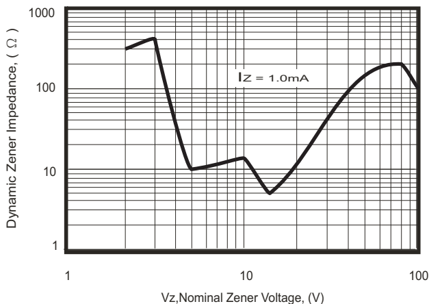
Fig.3- Zener Voltage vs Zener Impedance
