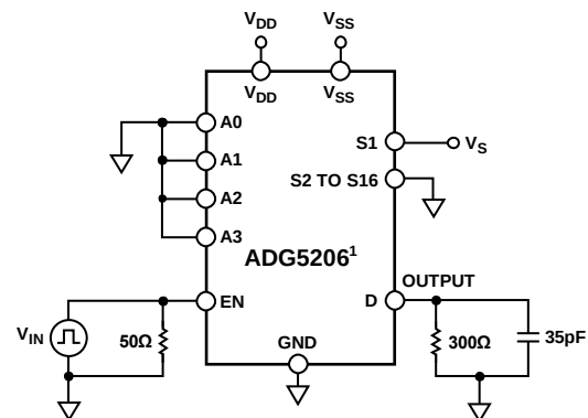
Figure 36. Enable Delay, t_{ON}(EN) , t_{OFF}(EN)
