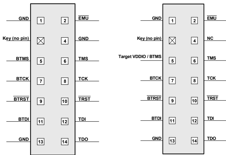
HPPCI JTAG I/O -- Legacy Pinout HPPCI JTAG I/O -- Auto Detection Pinout
