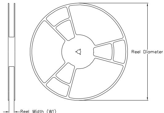
REEL DIMENSIONS
