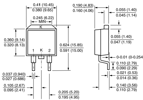
TO-263AB
