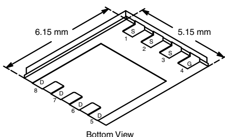
PowerPAK® SO-8
