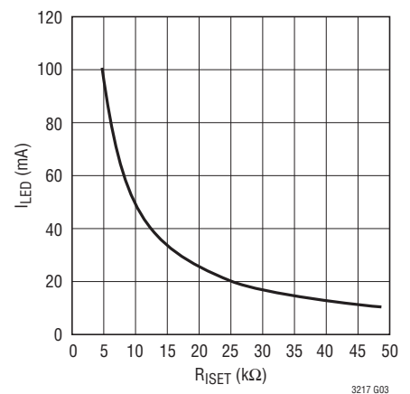
I_{\text{LED}} vs R_{\text{ISET}}
