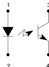
OPB315L
