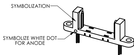
OPB315L
