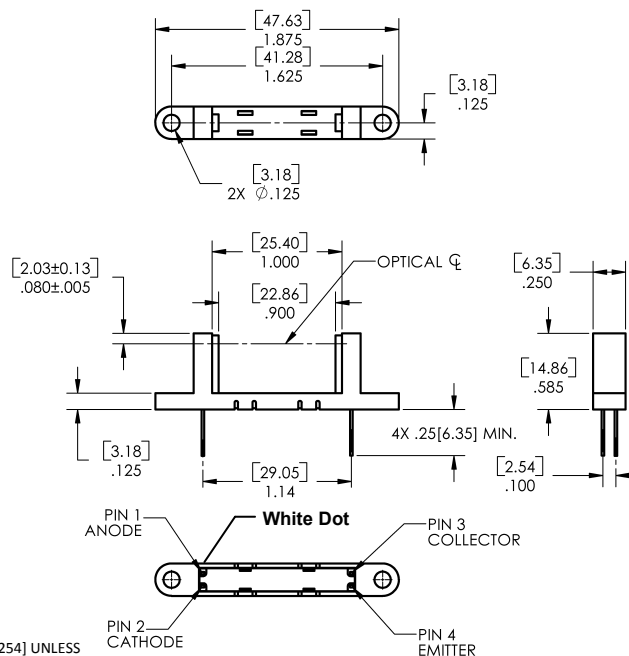
OPB315L
