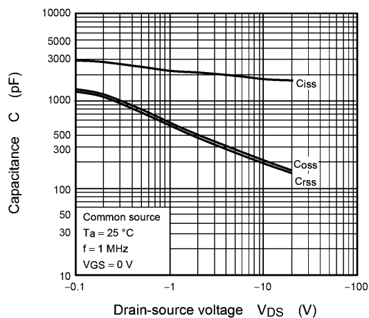
Fig. 7.9 C - V_{DS}
