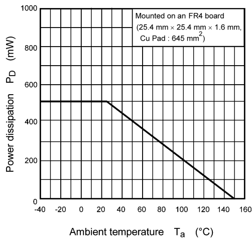
Fig. 7.13 P_D - T_a
