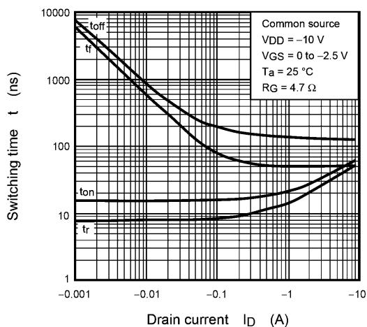
Fig. 7.10 t - I_D
