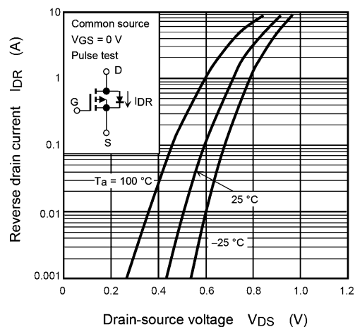
Fig. 7.8 I_{DR} - V_{DS}
