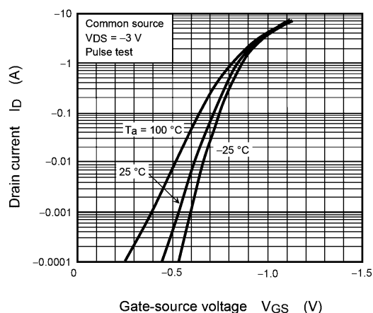
Fig. 7.2 I_D - V_{GS}
