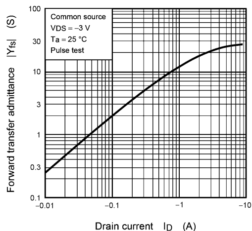
Fig. 7.7 |Y_{fs}| - I_D
