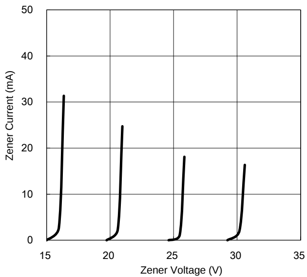
Zener Breakdown
