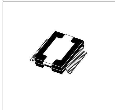
DIM. mm inch MIN. TYP. MAX. MIN. TYP. MAX. A 3.270 - 3.410 0.1287 - 0.1343 A2 3.100 - 3.180 0.1220 - 0.1252
