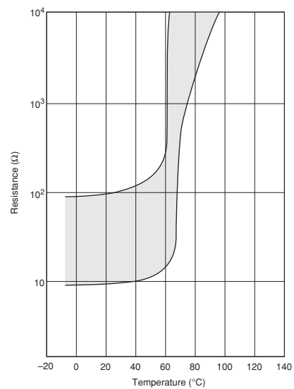
PTF_04BG471Q2N34B0
