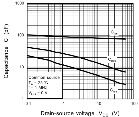
Fig. 7.8 C - V_{DS}
