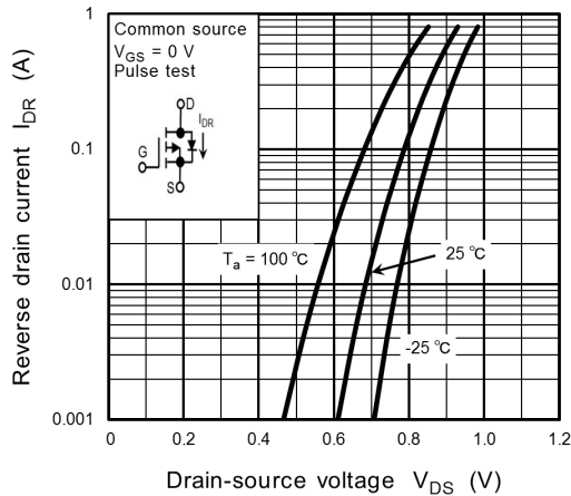
Fig. 7.7 I_{DR} - V_{DS}
