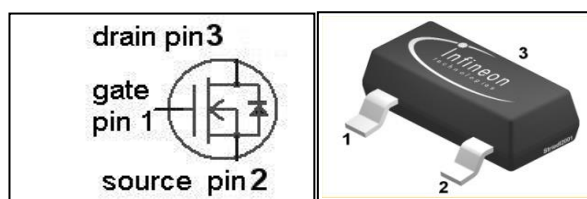
PG-SOT-23
