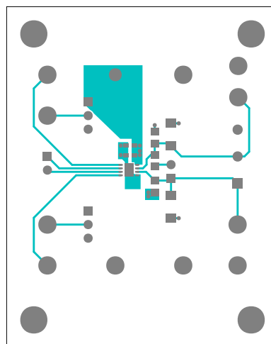
MAX14775E EV Kit—Top
