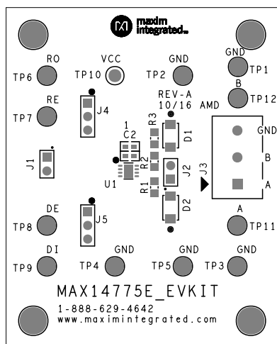
MAX14775E EV Kit—Top Silkscreen
