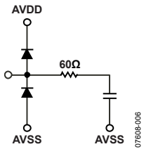
Figure 11. CCDIN (Pin 22)
