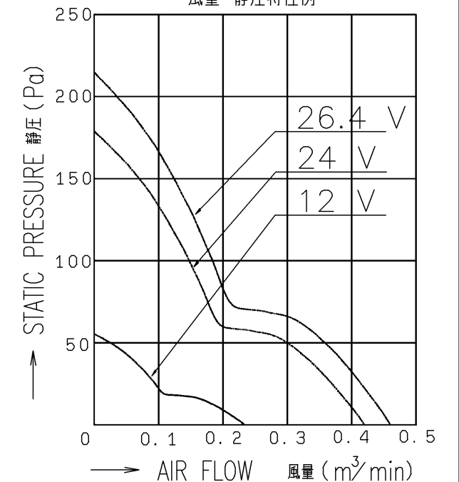
風量-靜壓特性例
