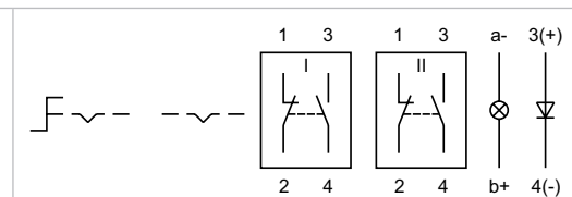
Wiring diagram 24
