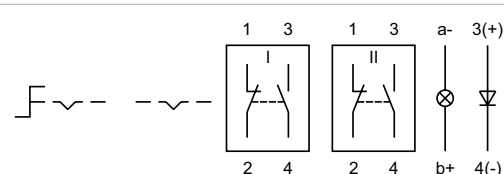
Wiring diagram 24
