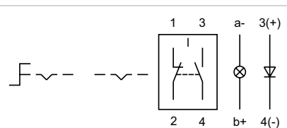
Wiring diagram 20
