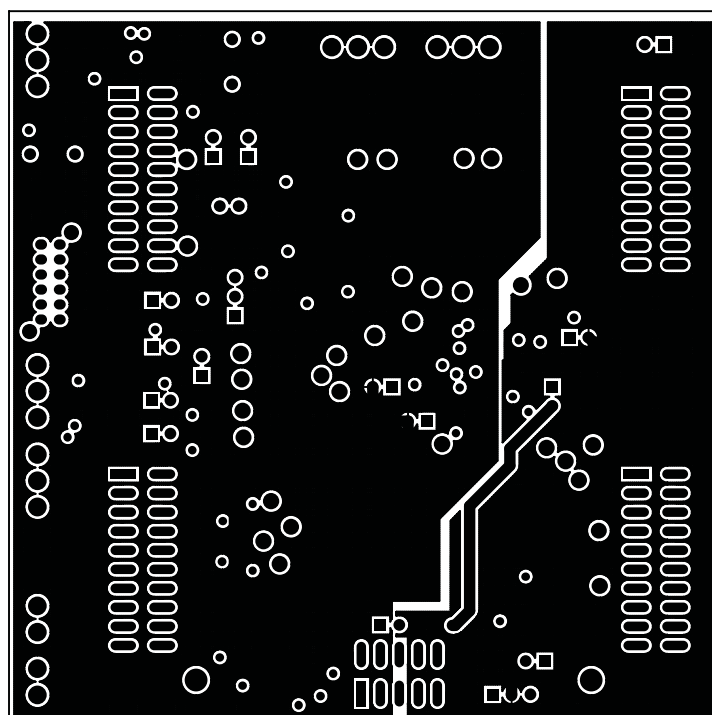
Figure C-4. Layer 4
