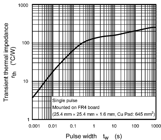
Fig. 7.13 r_{th} - t_w
