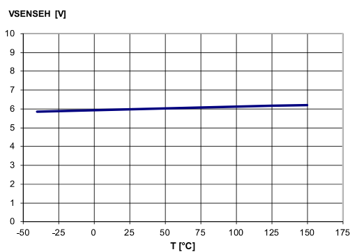
Figure 27: Vsenseh vs. Tcase
