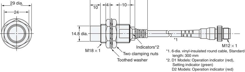
Diagram 32 E2E-X14MD□-M1GJ E2E-X14MD1-M1TGJ E2E-X14MD□-M1TGJ-US
