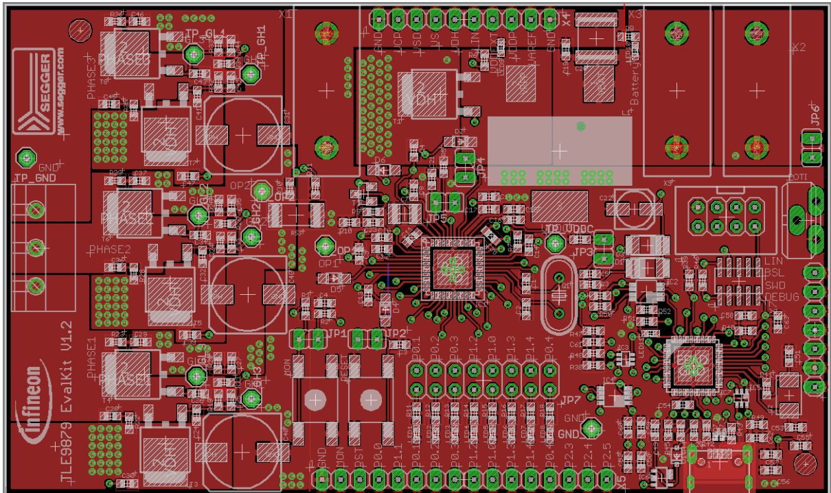
Top Layer
