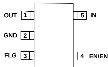
SOT25
