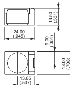
To fit round & Square bezel: A01FM2
