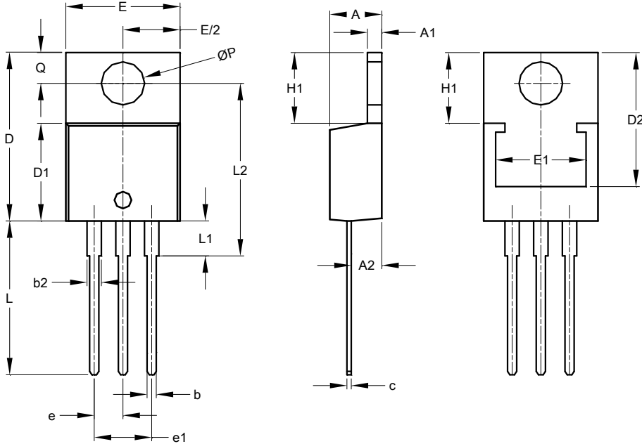
TO220AB
