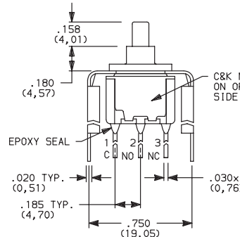
8121SD3_GE SPDT
