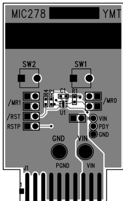
Top Layer
