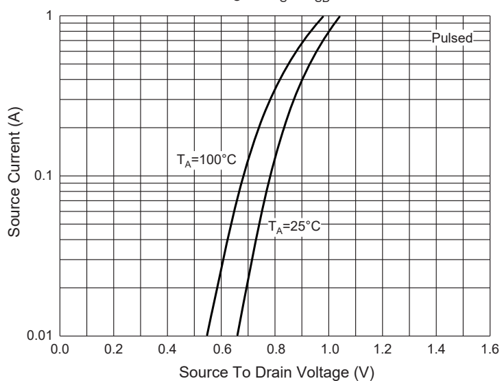
Fig. 5 - I_S - V_{SD}
