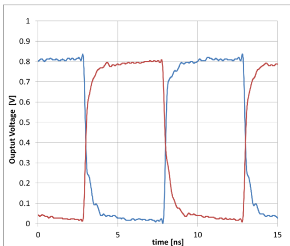
Figure 23. 100MHz HCSL
