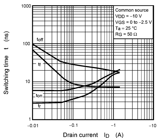
Fig. 7.11 t - I_D
