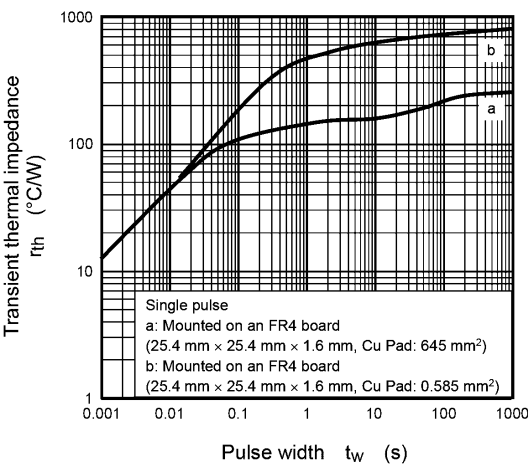
Fig. 7.13 r_{th} - t_w
