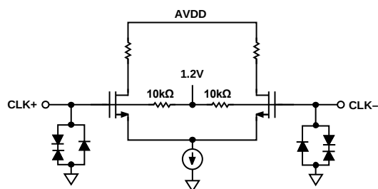
Figure 26. CLK± Inputs
