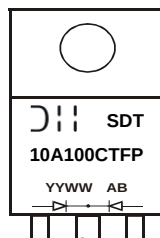
ITO220AB (Type HE)
